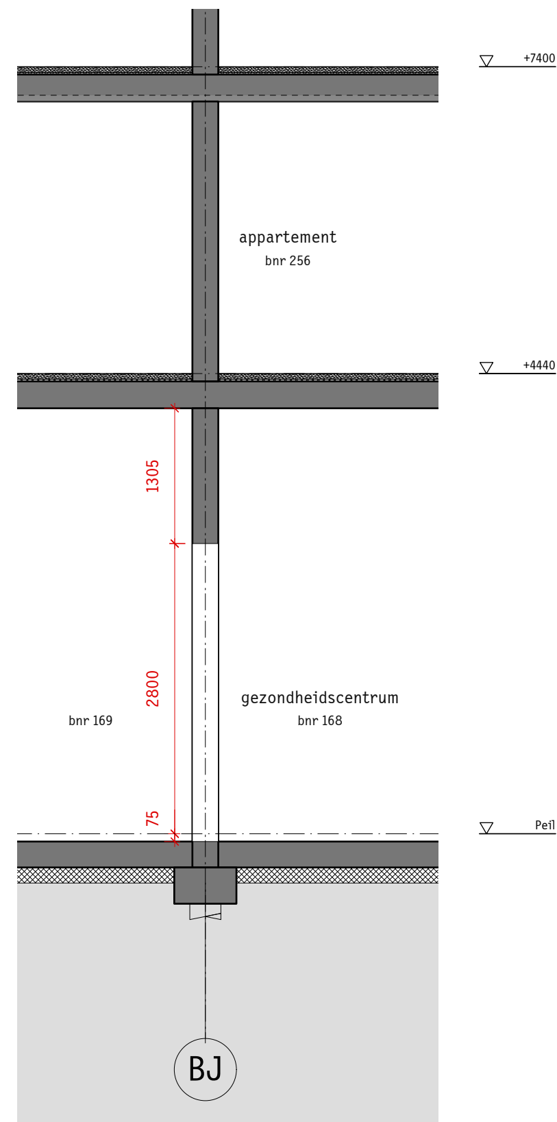
Doorsnede B
