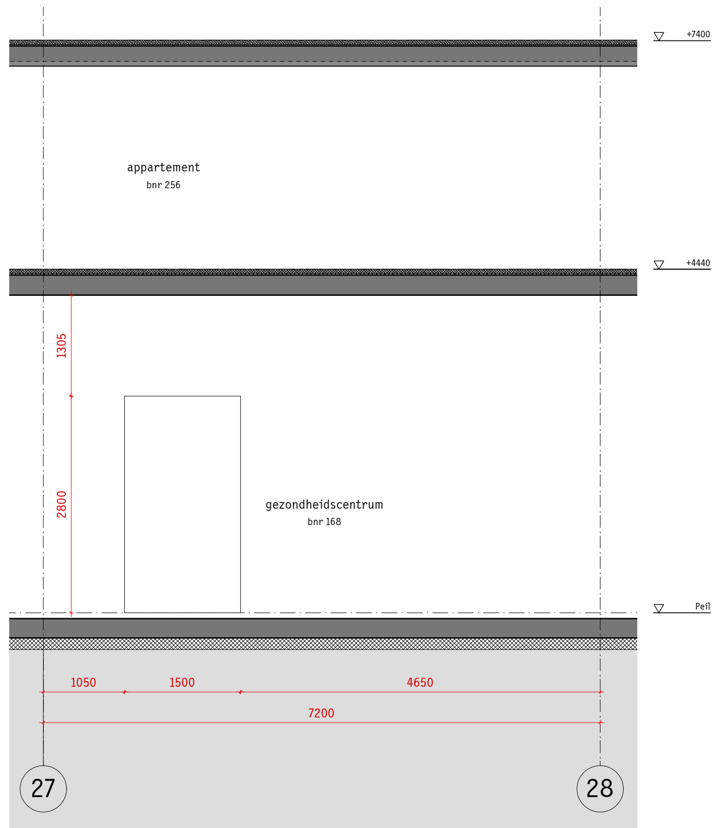
Doorsnede A
