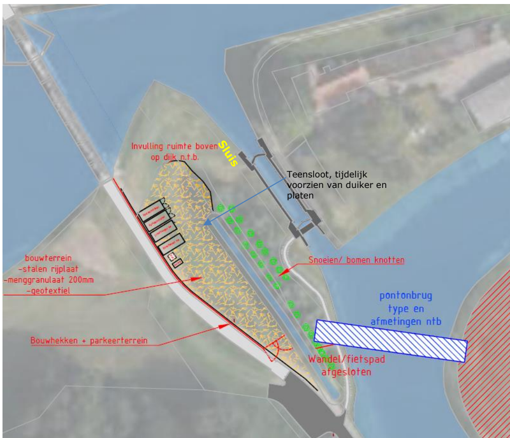
Figuur 6: Conceptindeling bouwterrein
