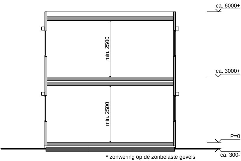
Dwarsdoorsnede
