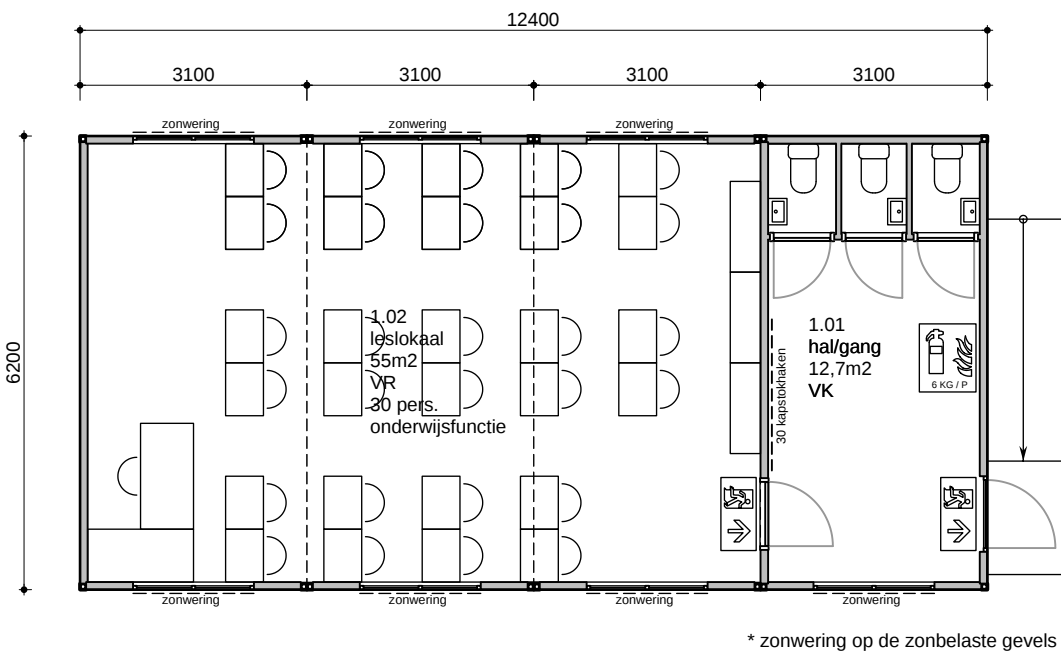
1e verdieping
