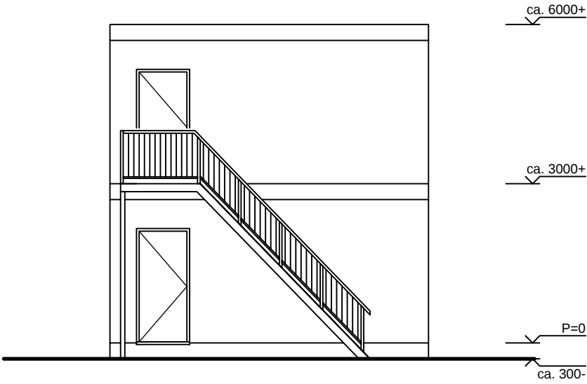
Rechter-zijgevel
